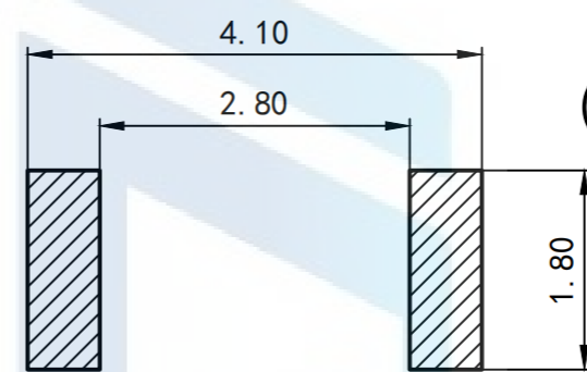
PCB. 焊接图
