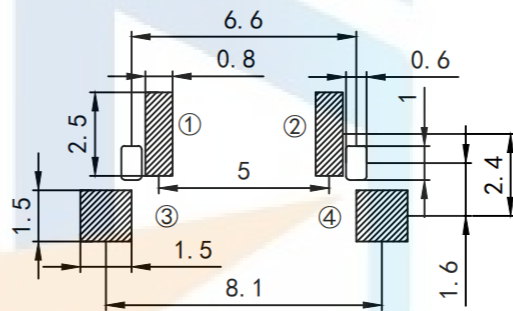
PCB. 焊接图
