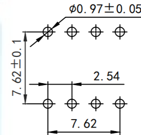
PCB开孔
